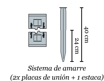
Sistema de amarre
